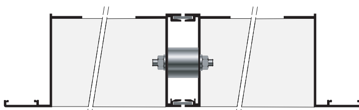
Gedeelde YGT over Nom. W voorzien van een dilatatievoeg
