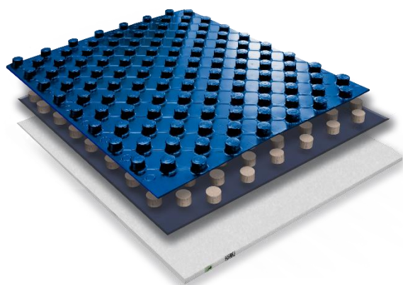
Figuur 2; 3D-weergave van de EnergyFloor
