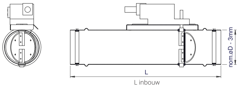
Tekening 3, doorsnede voor- en zij aanzicht WRS
