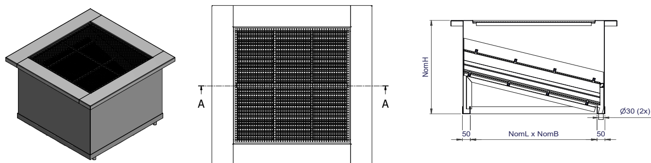
Tekening 4: AVDK - verzonken
