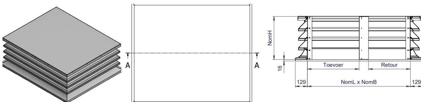
Tekening 2: ADK - Combi
