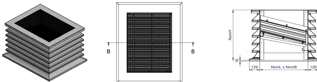
Tekening 3: AVDK
